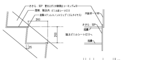
段部詳細図 1/10
