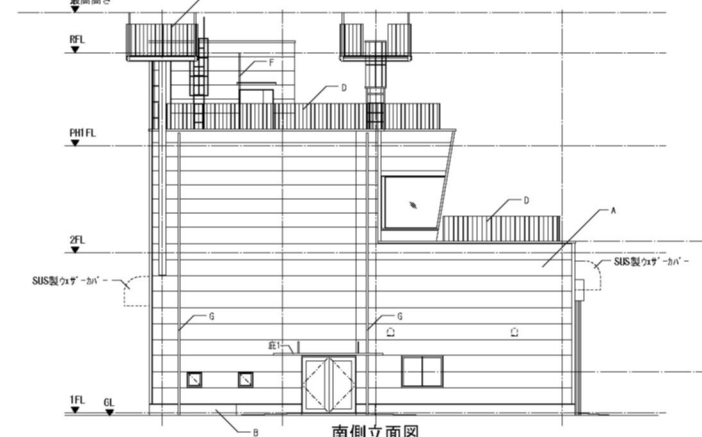
南側立面図
