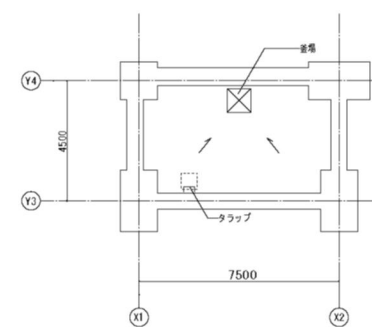
ビット伏図
