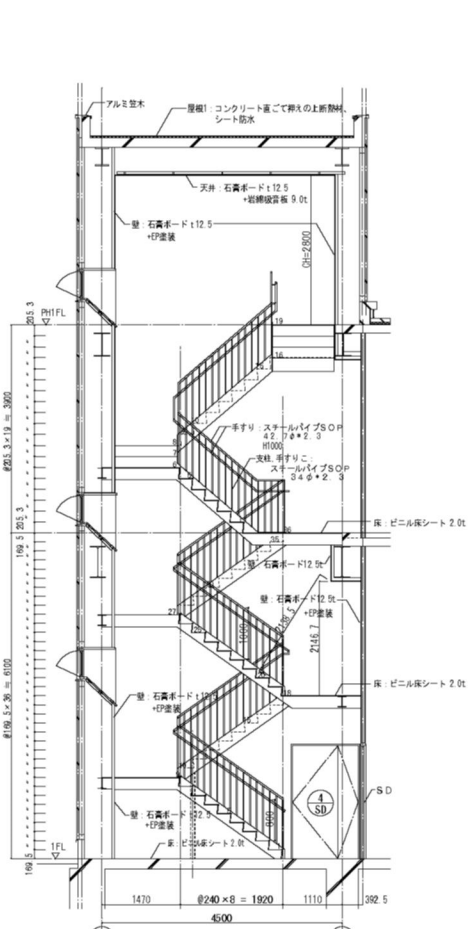
階段断面詳細図 1/50
