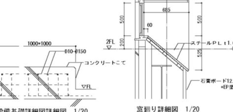
設備基礎詳細図 1/20
