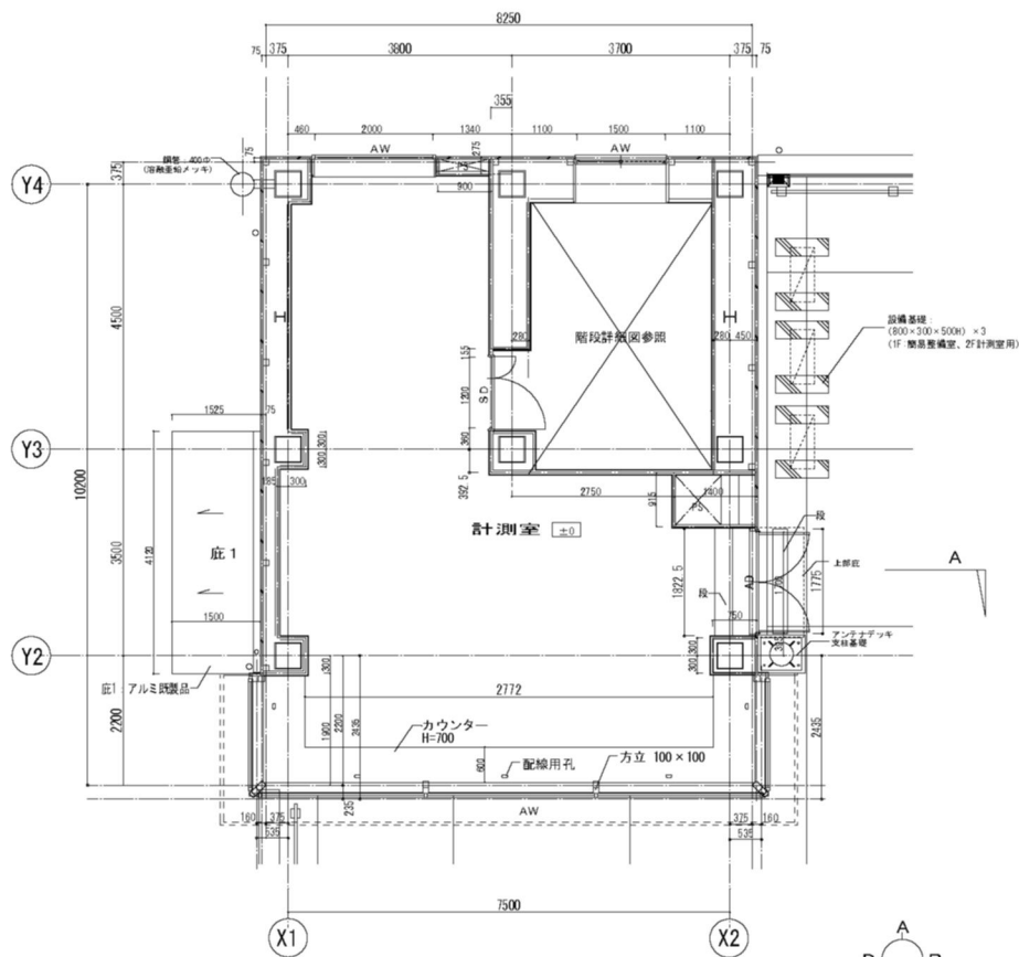
2階平面詳細図 1/50
