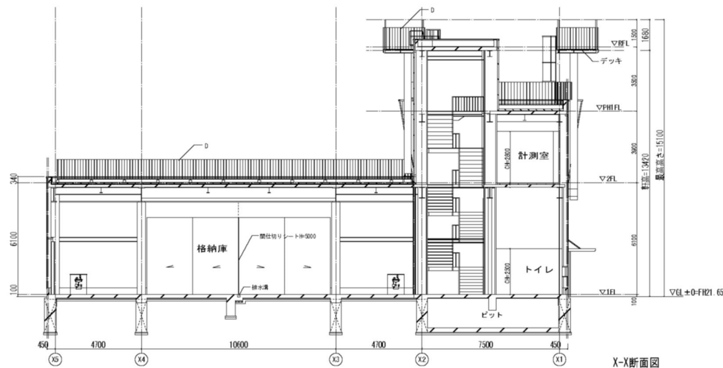
X-X断面図
