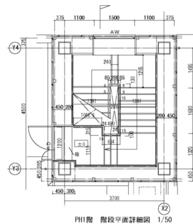
PH1階 階段平面詳細図 1/50
