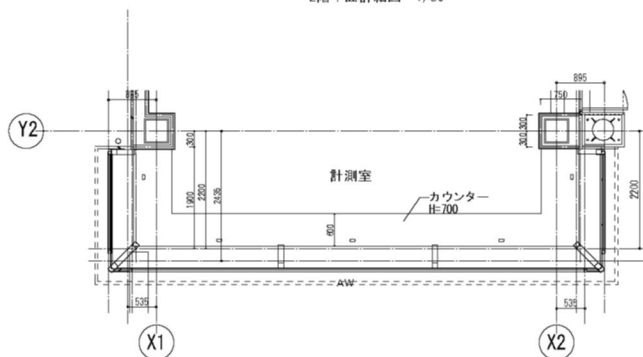
2階平面詳細図 (FL+2500) 1/50
