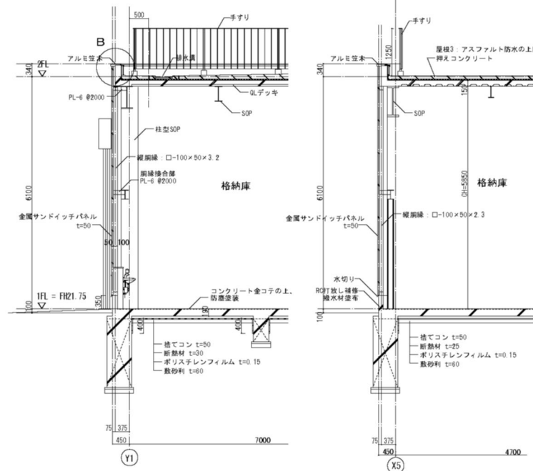
格納庫 1/50
