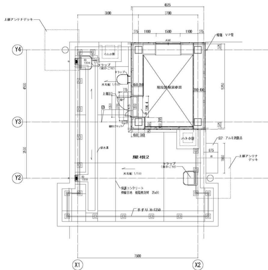
PH1階平面詳細図 1/50
