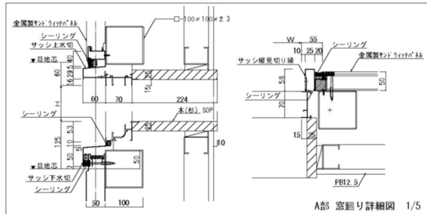
矩計図1 1/50
