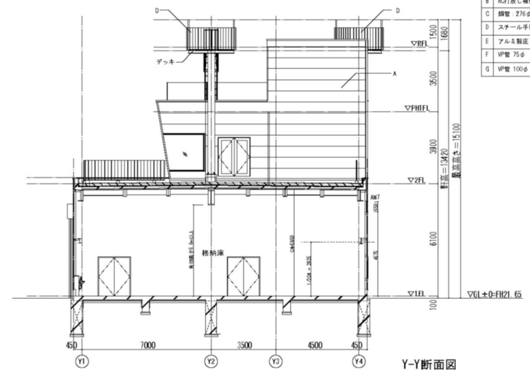
Y-Y断面図
