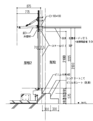
B断面詳細図 1/30 (A1)
