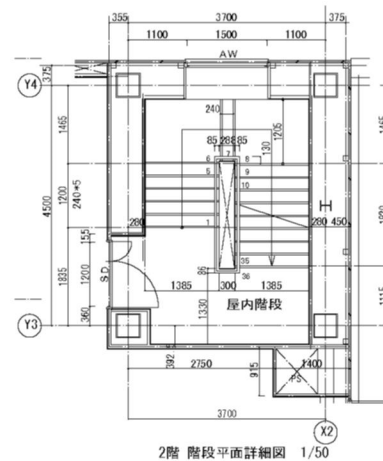
2階 階段平面詳細図 1/50
