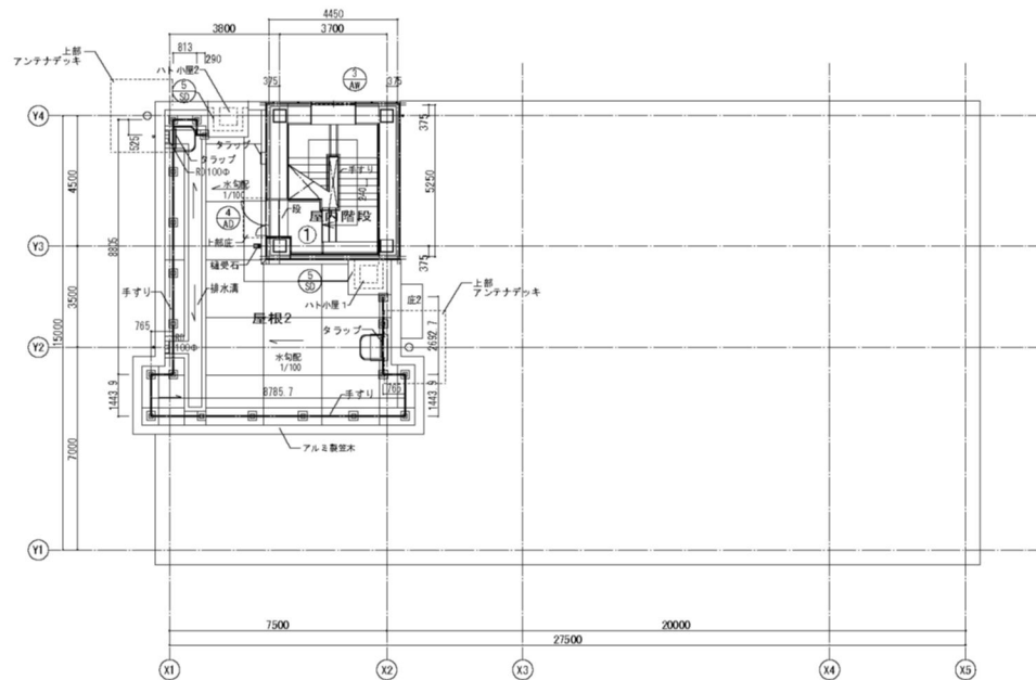
PH1階平面図
