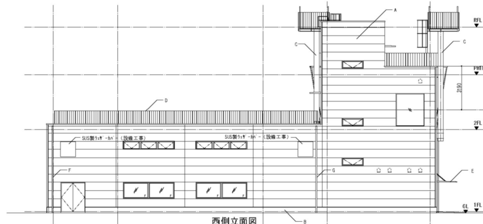
西側立面図
