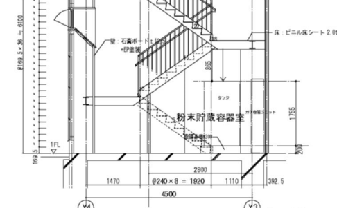
粉末貯蔵容器室断面詳細図 1/50
