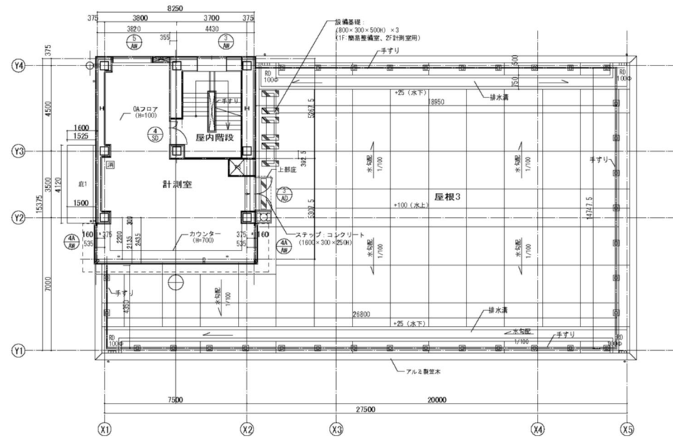
2階平面図
