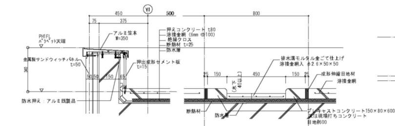
B部 バレータ立上り 詳細図 1/10
