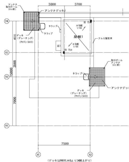
屋根伏図
