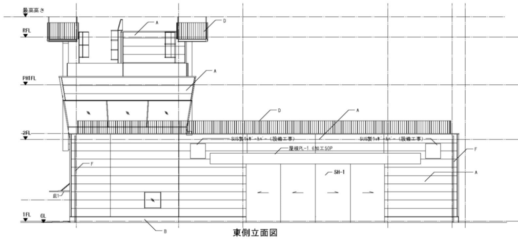
東側立面図
