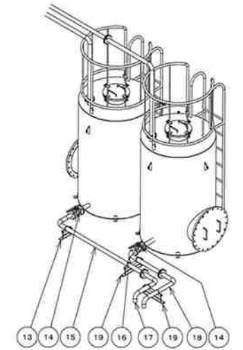
タンク裏面アイソメ図
